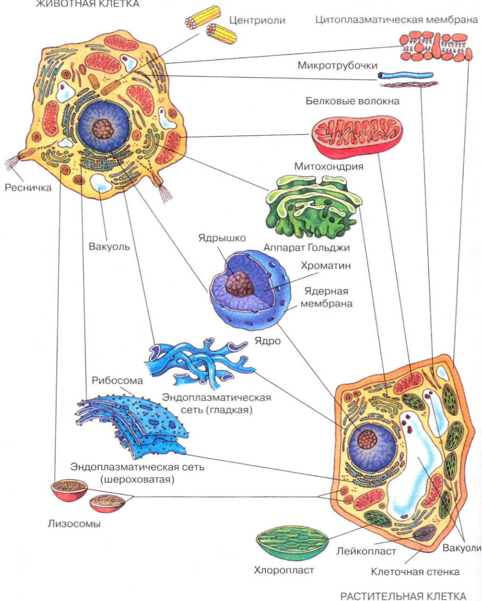
Рис. 68. Схема строения животной и растительной клеток
