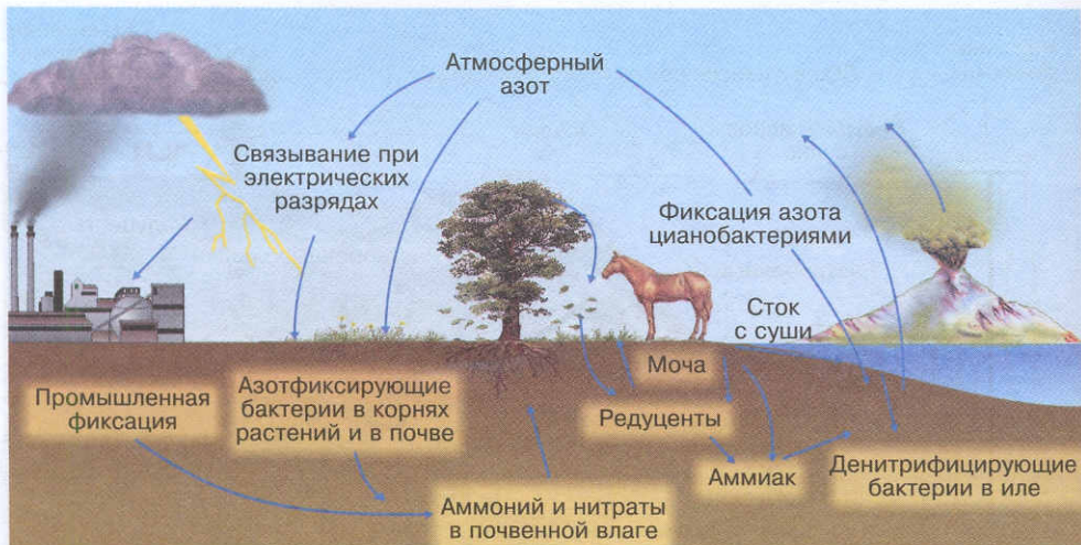
Рис. 119. Круговорот азота. Азот — один из важнейших компонентов белков и нуклеиновых кислот — генетического материала живых организмов
