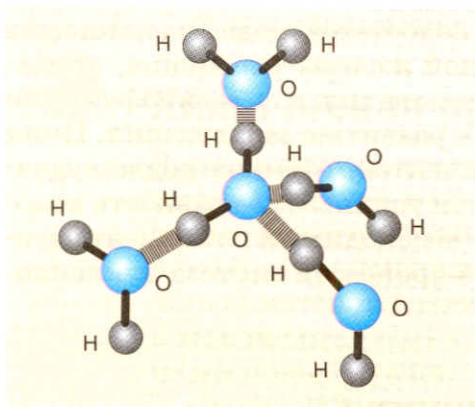
Рис. 59. Схема образования связей между отдельными диполями воды
