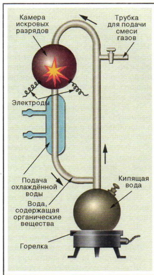
Рис. 115. Схема экспериментальной установки Г. Юри и С. Миллера для моделирования первичной атмосферы Земли
